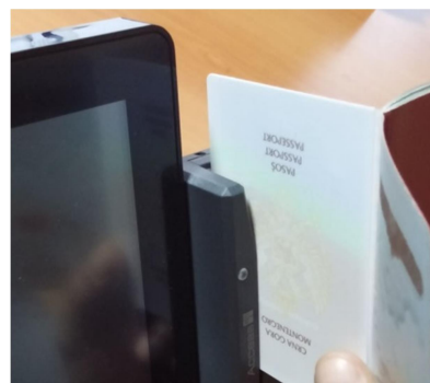
El. uređaj za identifikaciju birača i način provlačenja lične karte / pasoša kroz MRZ čitač
